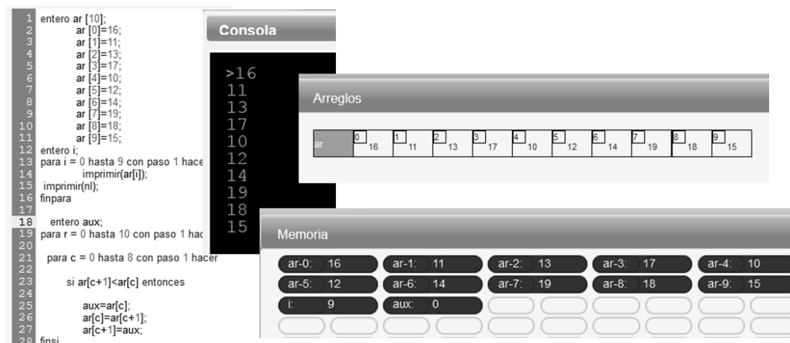
Fig. 6. Ejecución de un algoritmo en pseudocódigo y su representación gráfica.
