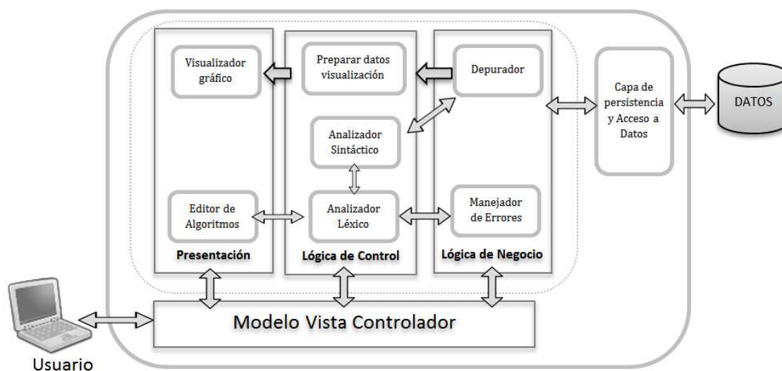
Fig. 2. Diagrama general de la herramienta.
