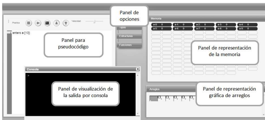
Fig. 3. Área de trabajo de la herramienta.
