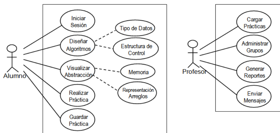
Fig. 1. Diagrama de casos de uso de la herramienta didáctica.
