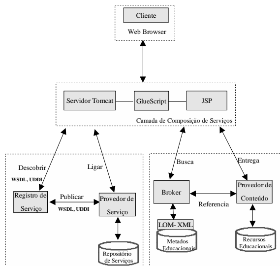
Figura 2: Protótipo da Arquitetura da DSL GlueScript [Hansen 2003]
