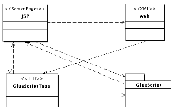
Figura 3: Diagrama UML da GlueScript
