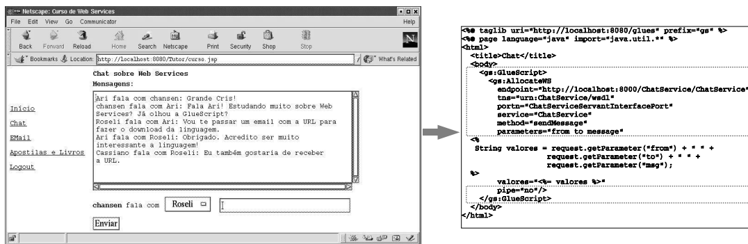
Figura 9: Página de Chat do Curso
