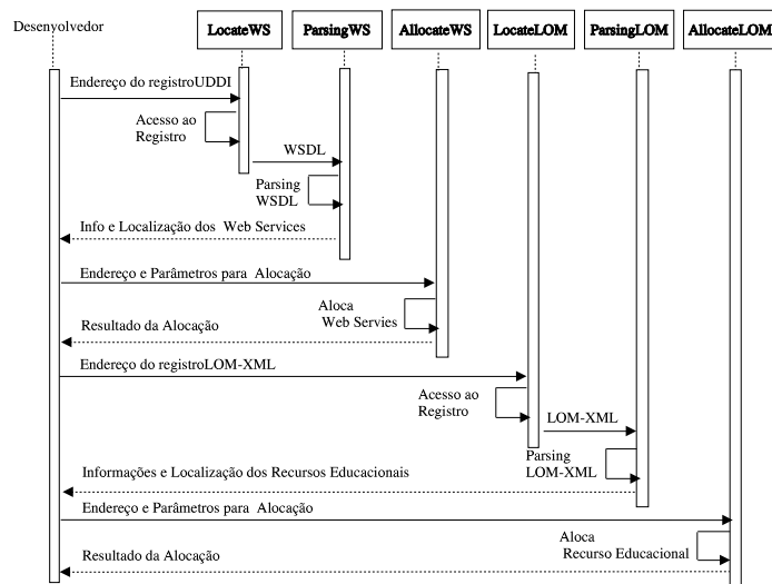
Figura 5: Diagrama de Sequência das Tags da GlueScript
