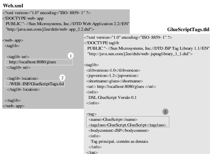
Figura 4: Relacionamento dos Arquivos web.xml e GlueScriptTags.tld
