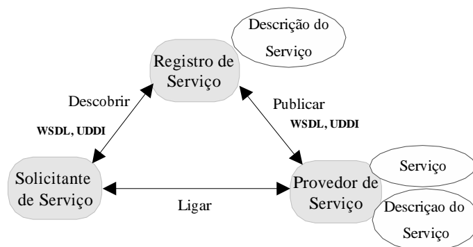
Figura 1: Web Services Papéis, Operações e Artefatos [ Kreger 2001]
