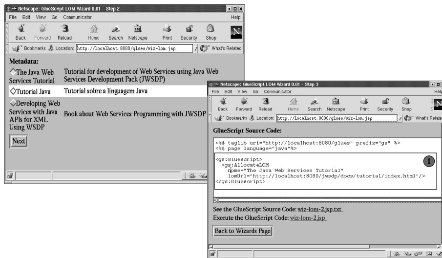
Figura 7: Assistente GlueScript - Escolha do Recurso e Geração do Código
